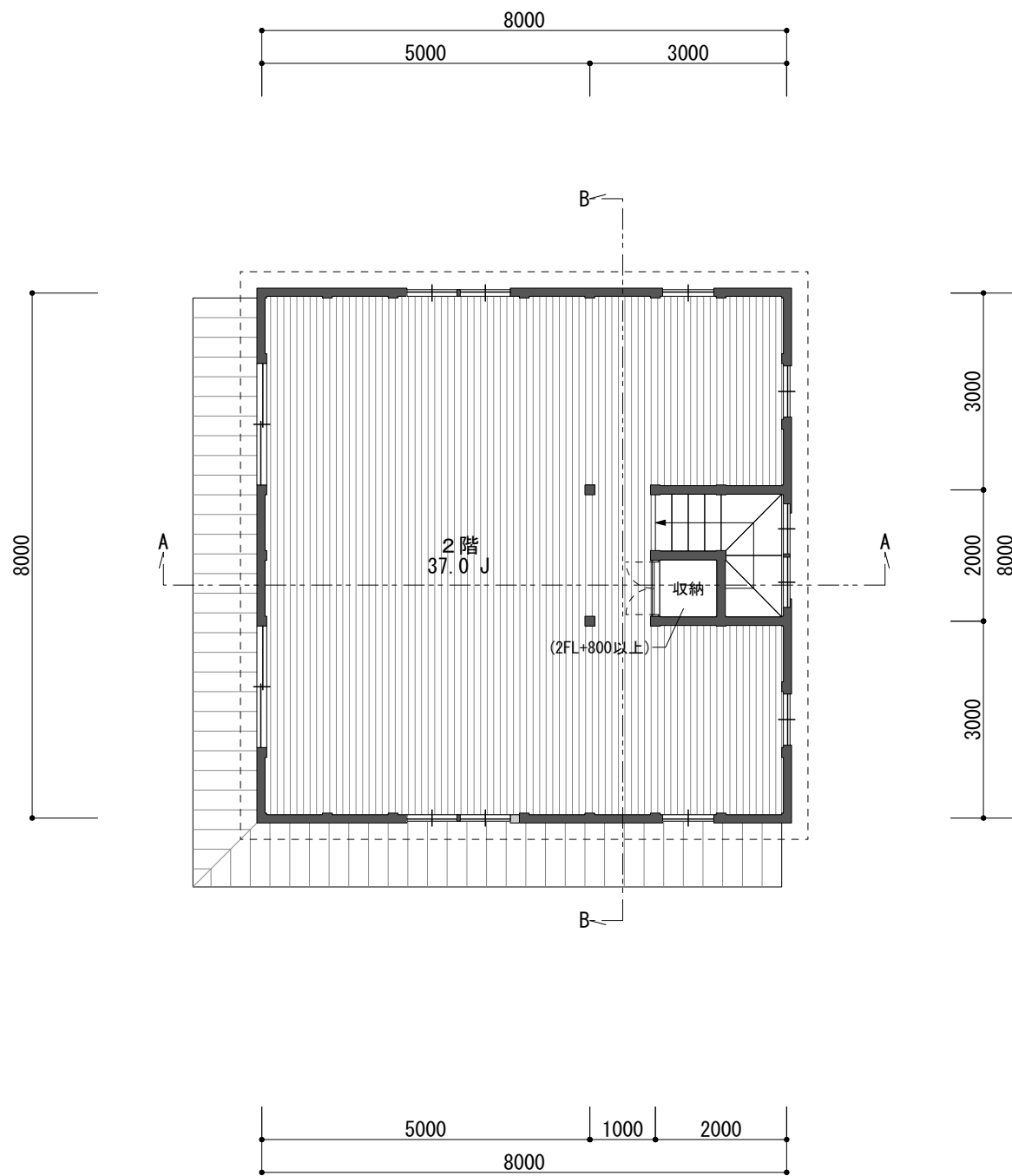
2階平面図
