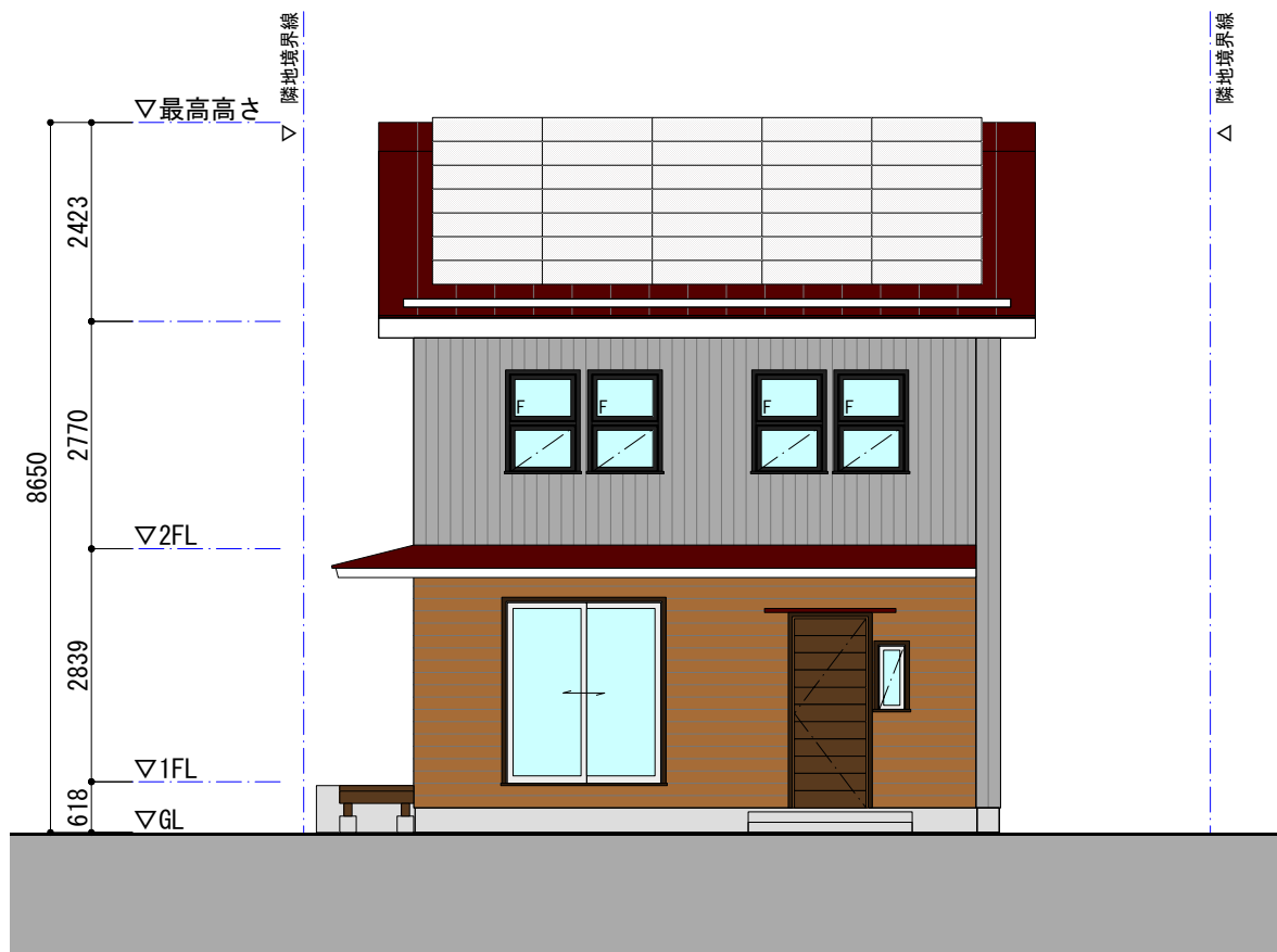
南側立面図
