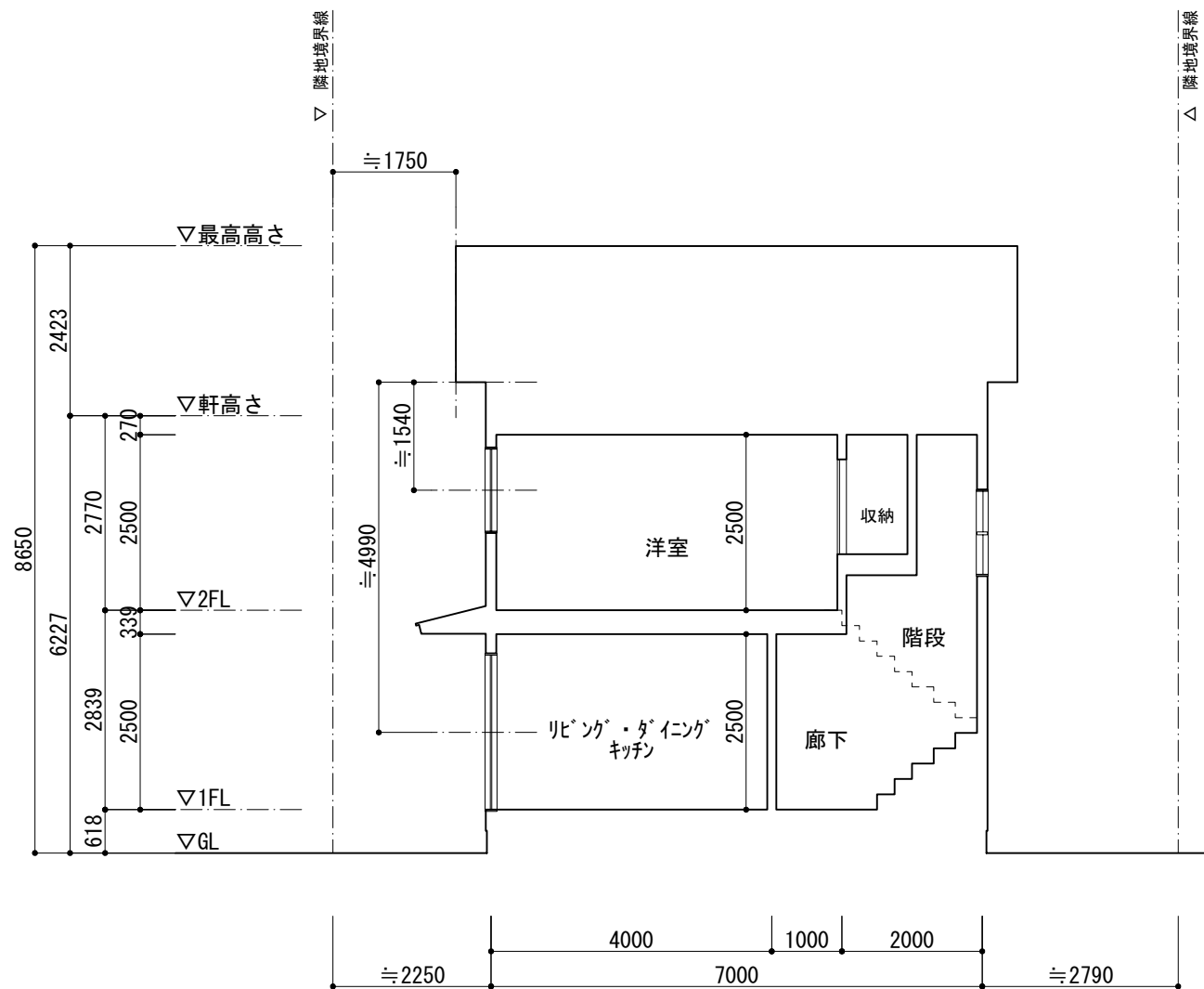
A-A 断面図
