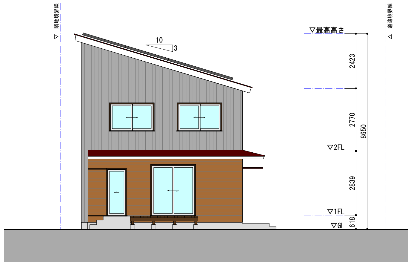
西側立面図
