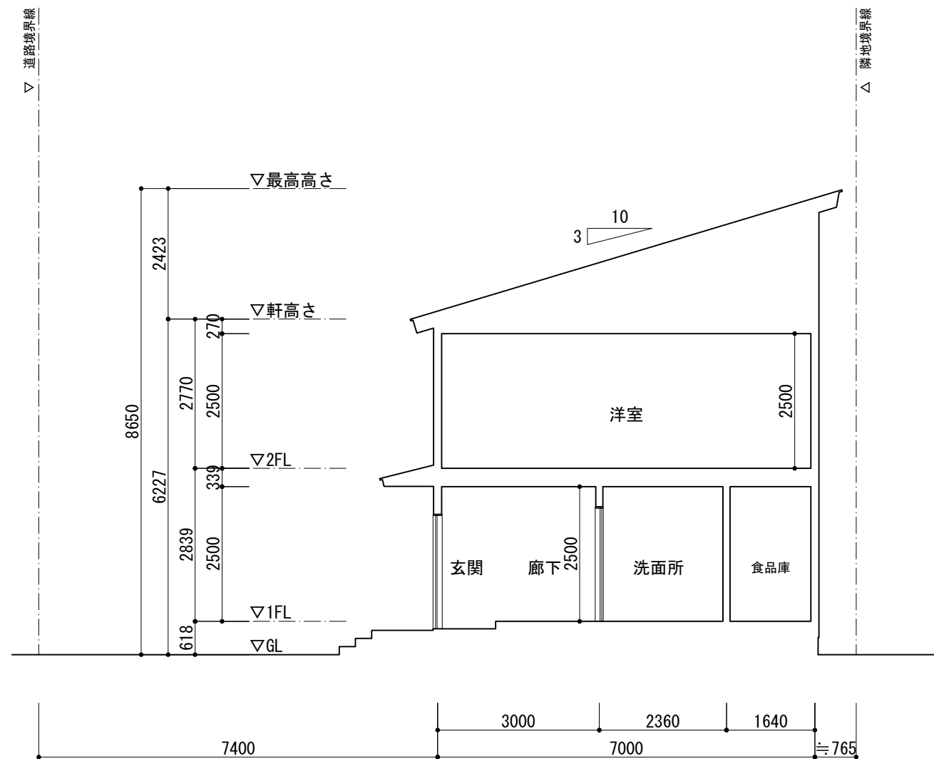
B-B 断面図
